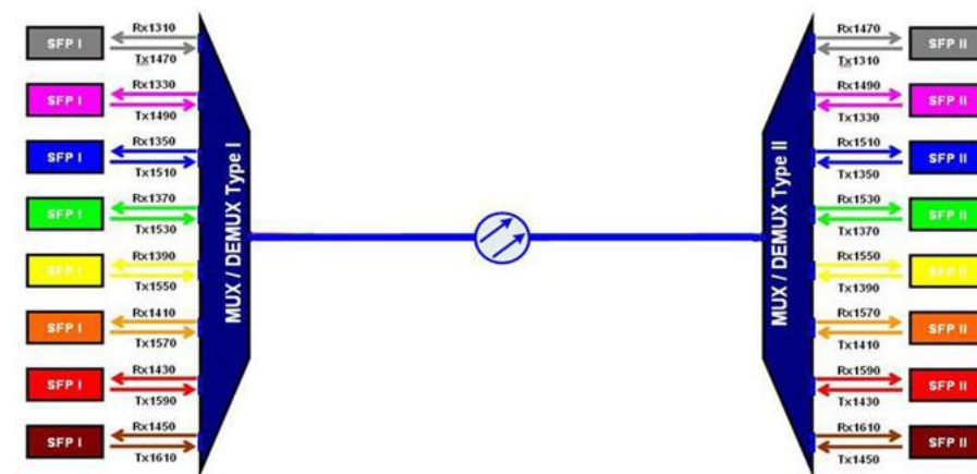
DWDM
